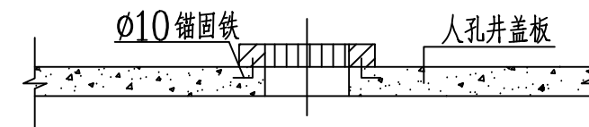
1—1 剖面
