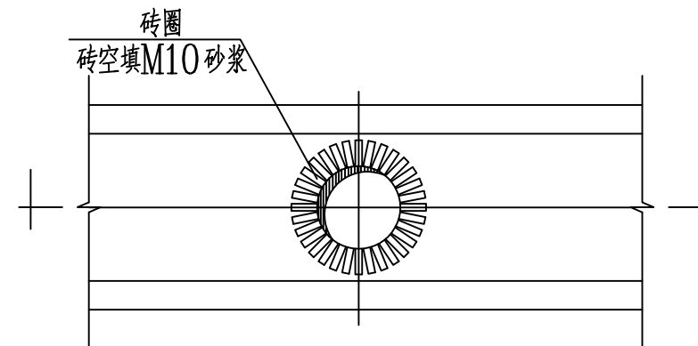
井盖口圈砖砌图
