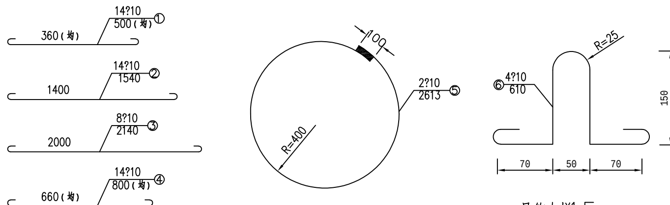
吊钩大样1:5
