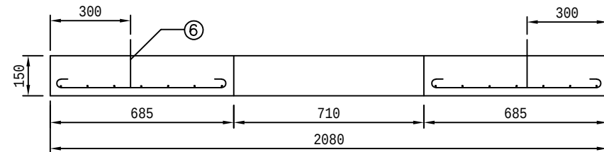
I—I 剖面图1:20
